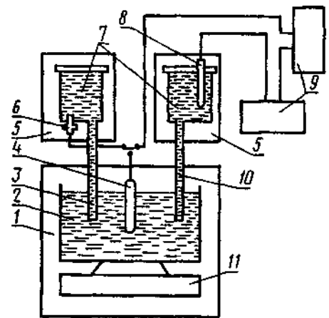
Схема установки для определения потенциала электродов
